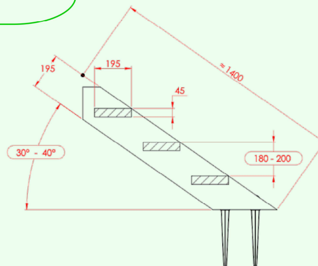
COUPE A-A
